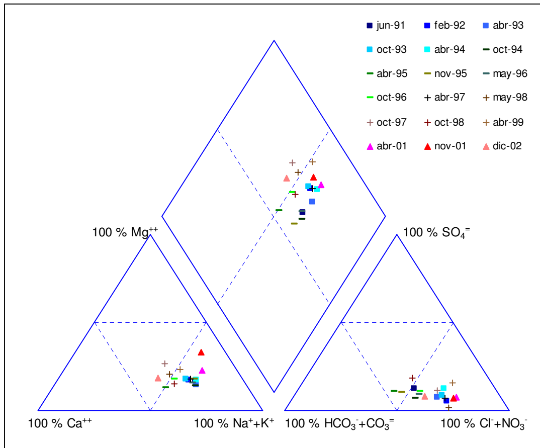
Fig. 3 Diagrama de Piper-Hill-Langelier de la captación nº 114150061.
