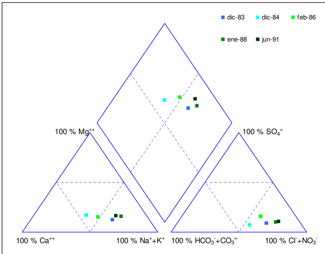
Fig. 4 Diagrama de Piper-Hill-Langelier de la captación nº 1141510063.
